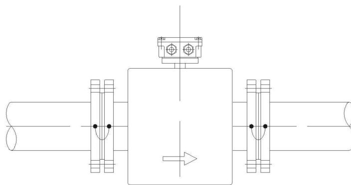
a) rurowciąg metalowy z kołnierzami elektrycznie izolowanymi od rurowciągu
