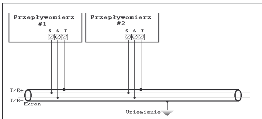
Rys.3 Podłączenie do istniejącej sieci
