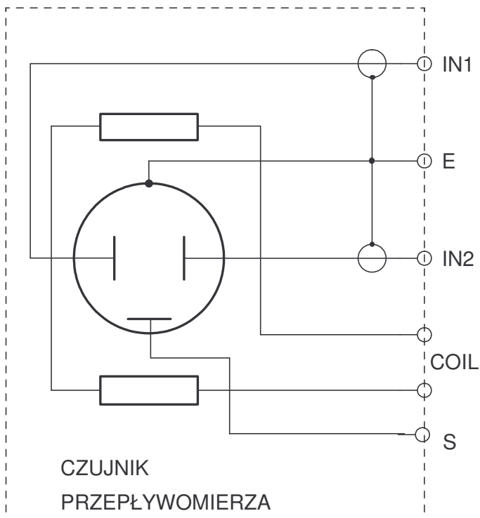
Rys. 6b. Połączenia zewnętrzne czujnika i przetwornika (w wykonaniu z czujnikiem pustej rury ERP).
