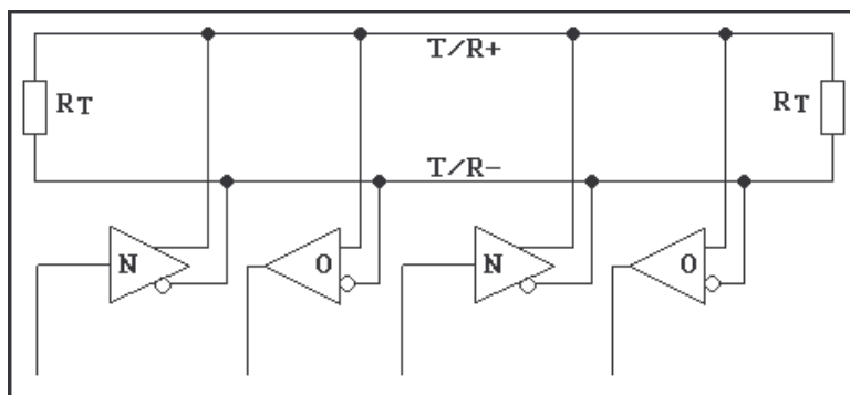
Rys.1 Rezystory dopasowujące R_T
