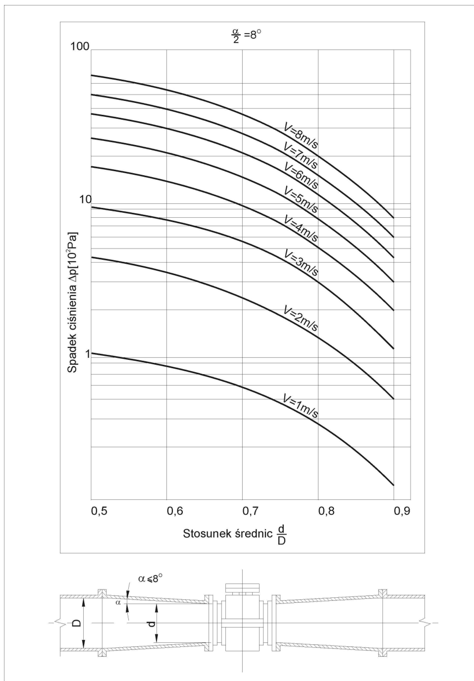
rys.2 Spadek ciśnienia na czujniku
