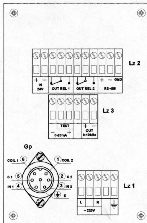
Rys.6. Schemat połączeń czujnika i przetwornika typu MPP-04 T
