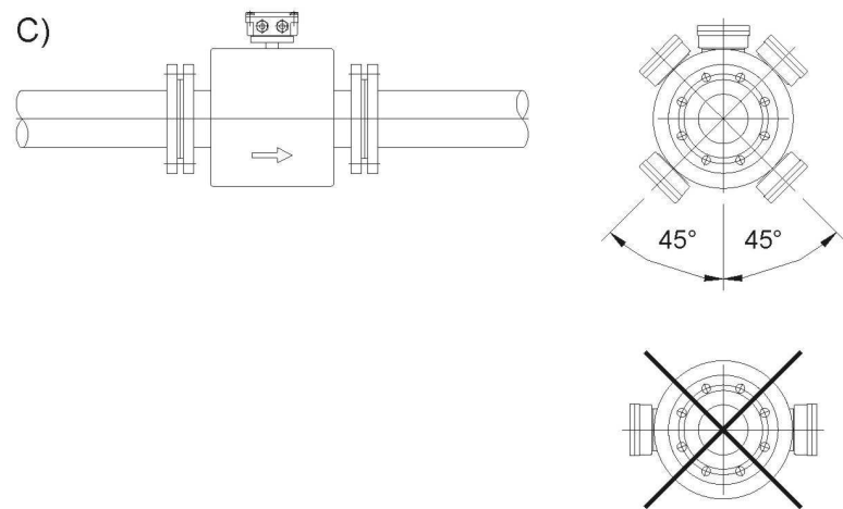
Rys.3. Montaż czujnika
