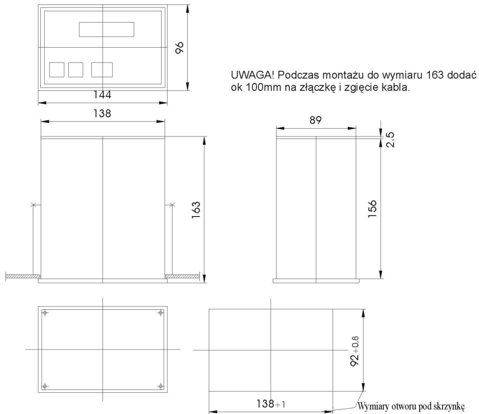
Rys.5. Wymiary zewnętrzne przetwornika
