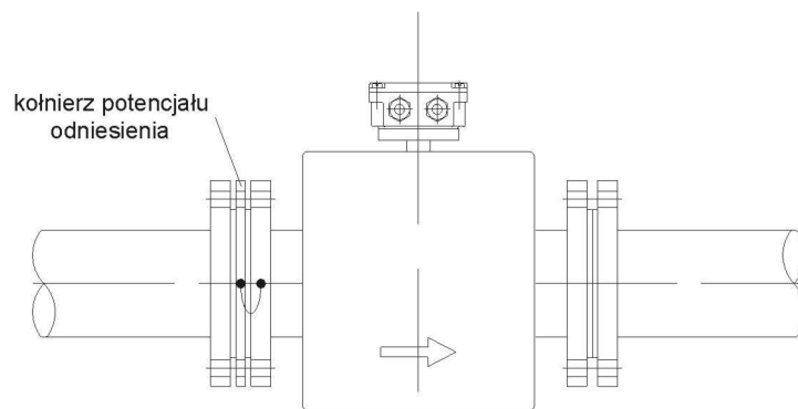
b) rurowciąg z kołnierzami metalowymi
