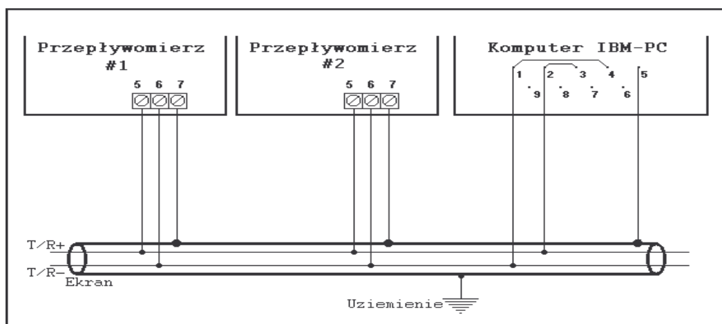
Rys.2 Połączenia interfejsu sieciowego
