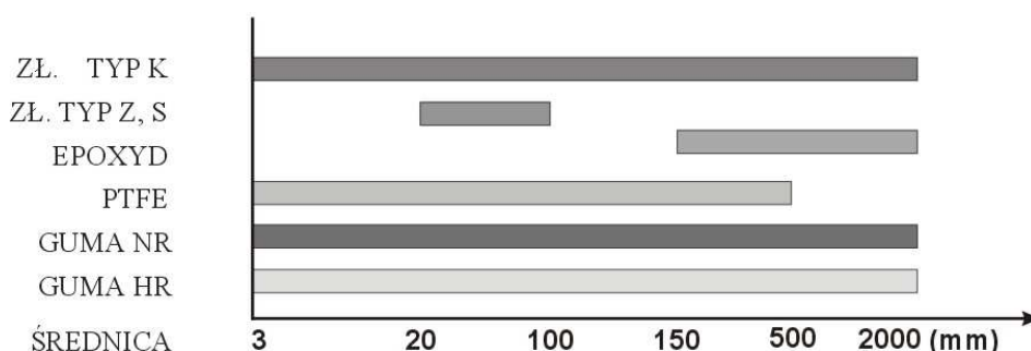
Wykres nr 1. Typy złącz i wykładzin dostępnych dla danej średnicy czujnika.
